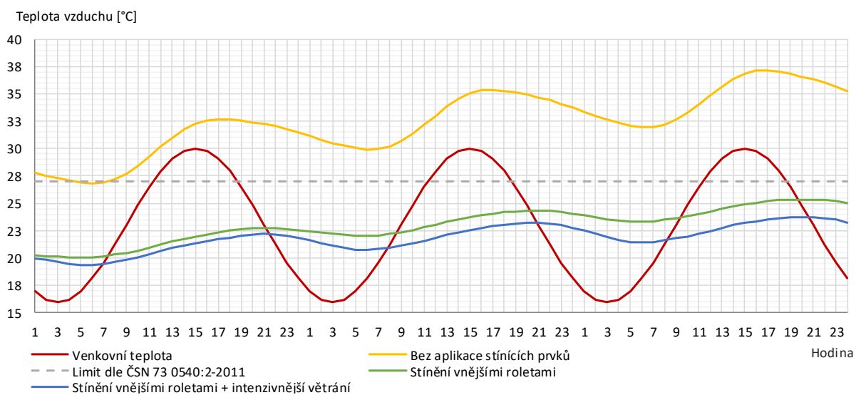
Obrázek 31 Modelové zobrazení efektu použití vnějších stínících prvků na vnitřní teplotu v objektu (zdroj: PORSENNA o.p.s.)
