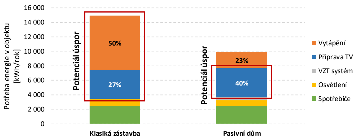
Obrázek 33 Porovnání rozložení potřeby energie v klasické zástavbě / pasivním domě (PORSENNA o.p.s.)
